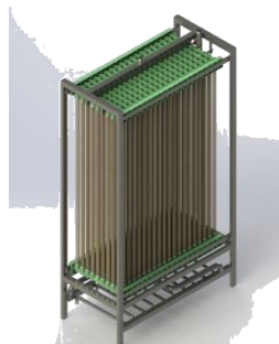
Megaflux-MBR 침지식 프레임 Megaflux-MBR submerged frame
